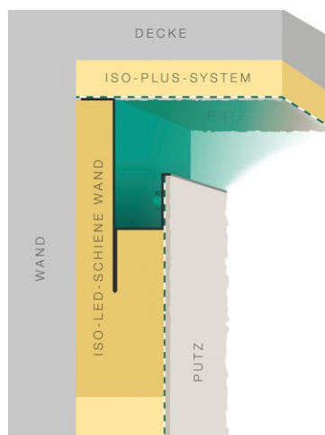
Spezielle Eck-Elemente je nach Einbau-Situation
